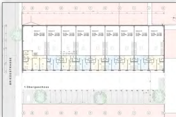
Grundriss 1.OG
