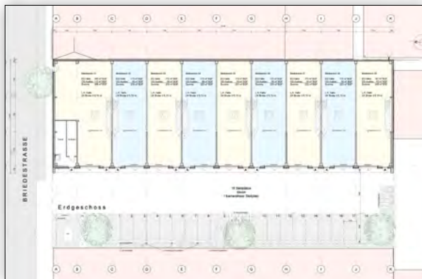
Grundriss EG
